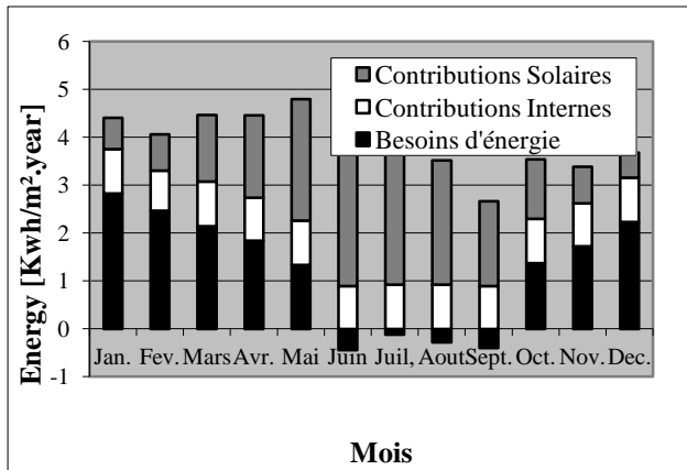
Figure 8: Relation entre les besoins énergétiques, les apports internes et solaires [6]
